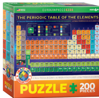
The Periodic Table
